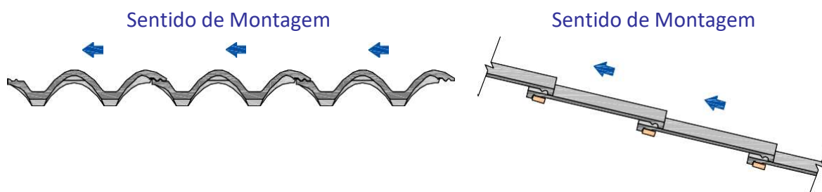
Figura 5 – Seqüência de montagem das telhas
