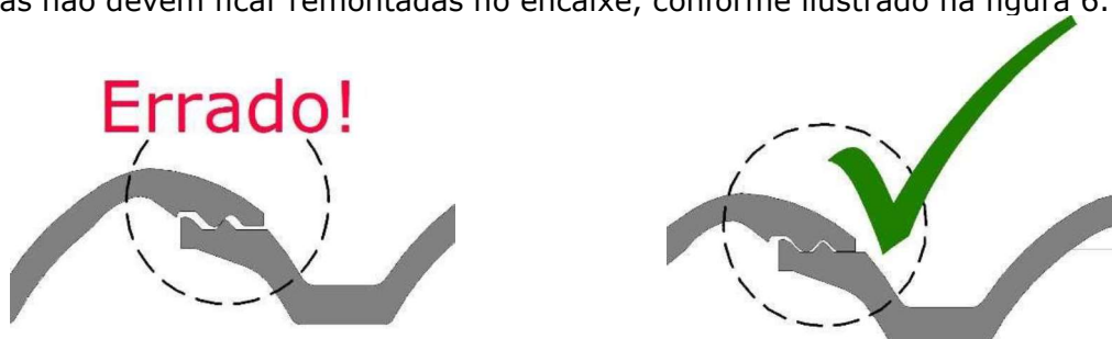
Figura 6 – Ajuste da telha
