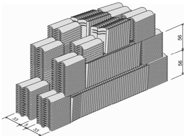
Figura 4 – Forma de empilhamento das telhas na obra
